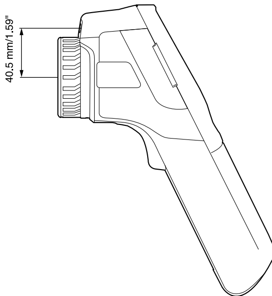
図 6.1 この図は、レーザー ポインタと赤外線レンズの光心の間にある位置の違いを示しています。
