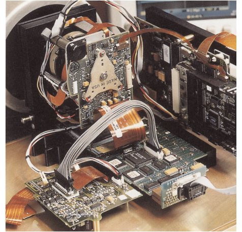
図 25.3 左: システムエレクトロニクスの開発。右: FPA 検出素子のテスト
