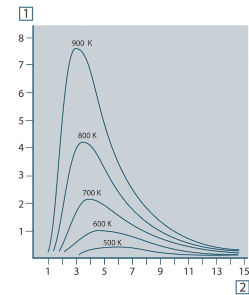
図 29.4 Planck の法則に従ってさまざまな絶対温度に対して描画された黒体スペクトル放射発散度。1 : スペクトル放射発散度 (W/cm 2 × 10 3 (μm))、2 : 波長 (μm)
