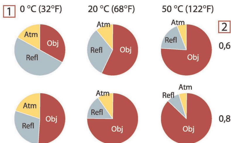
図 30.2 変化する測定条件下での放射線源の相対的な大きさ (SW カメラ)。1: 対象物の温度、2: 放射率、Obj: 物体放射、Refl: 反射放射、Atm: 大気放射。固定パラメータ: \tau = 0.88 , T_{\text{refl}} = 20^{\circ}\text{C} , T_{\text{atm}} = 20^{\circ}\text{C} 。
