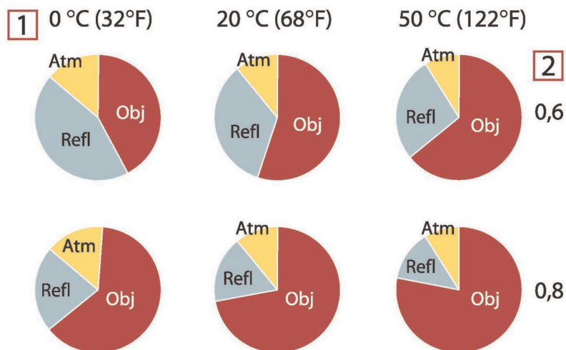
図 30.3 変化する測定条件下での放射線源の相対的な大きさ (LW カメラ)。1: 対象物の温度、2:放射率、Obj: 物体放射、Refl: 反射放射、Atm: 大気放射。固定パラメータ: \tau = 0.88 、 T_{\text{refl}} = 20^\circ\text{C} 、 T_{\text{atm}} = 20^\circ\text{C} 。
