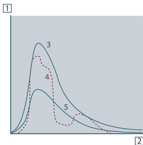
図 29.8 3 種類の放射体の分光放射率。1：分光放射率、2：波長、3：黒体、4：選択放射体、5：灰色体。
