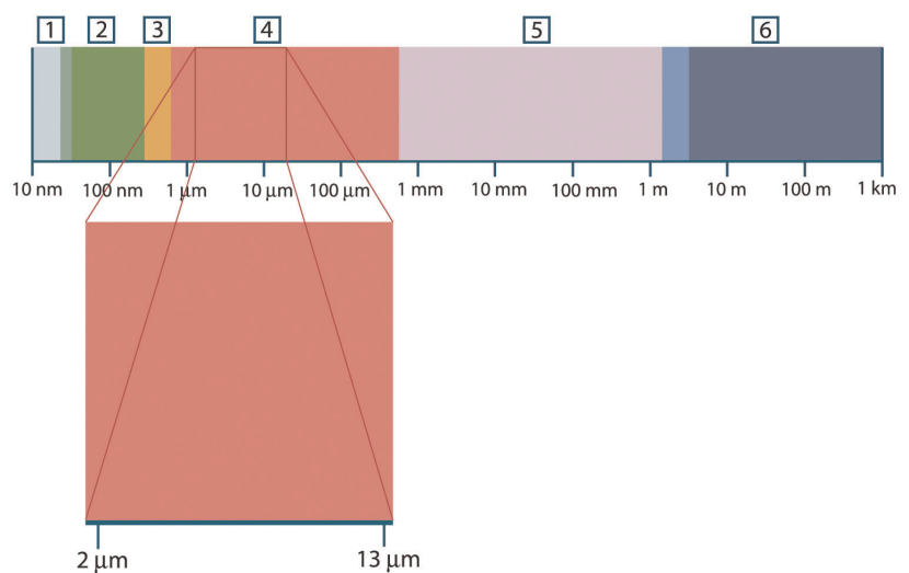
図 29.1 電磁スペクトル。1：X 線、2：紫外線、3：可視光、4：赤外線、5：マイクロ波、6：電波。
