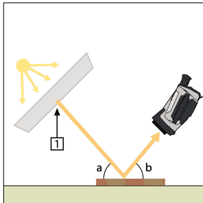
図 27.2 1 = 反射源
