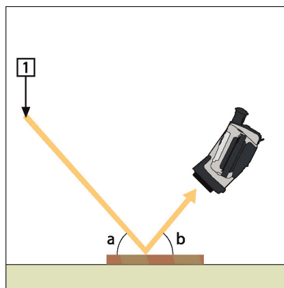
図 27.1 1 = 反射源
