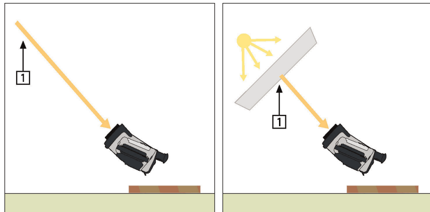
図 27.3 1 = 反射源
