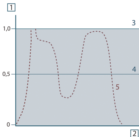
図 29.9 3 種類の放射体の分光放射率。1：分光放射率、2：波長、3：黒体、4：灰色体、5：選択放射体。
