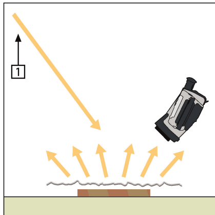
図 27.4 アルミホイルの見かけ温度を測定します。
