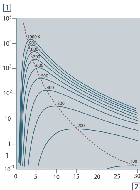
図 29.6 100 K から 1000 K までの半対数目盛で描画された Planckian の曲線。点線は、Wien の変位の法則で説明した各温度での最大放射発散度の軌跡を表しています。1：スペクトル放射発散度 ( \text{W}/\text{cm}^2 ( \mu\text{m} )), 2：波長 ( \mu\text{m} )。
