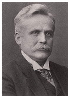
図 29.5 Wilhelm Wien (1864 ~ 1928)
