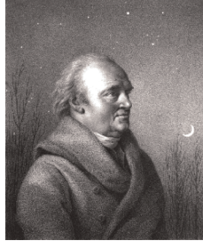
図 28.1 William Herschel 卿 (1738–1822)
