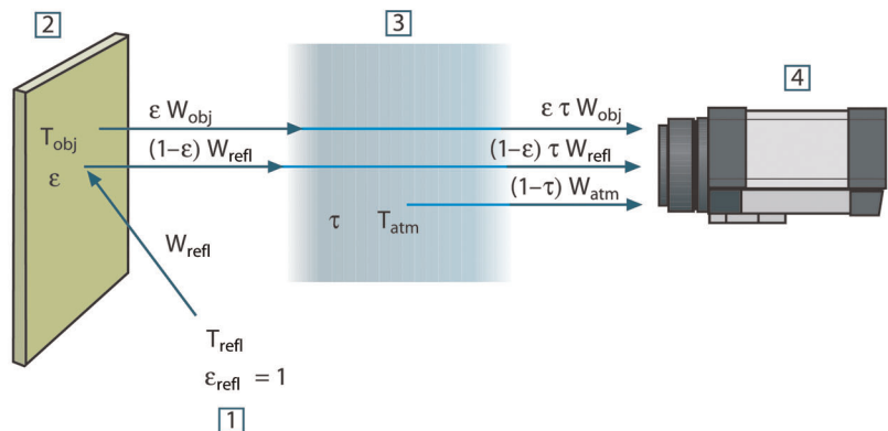
図 30.1 一般的なサーモグラフィ測定状態の図式表示。1：周囲、2：物体、3：大気、4：カメラ
