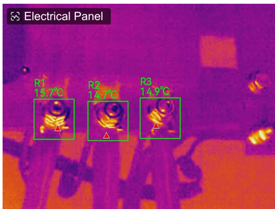
図5-2 電気パネル
