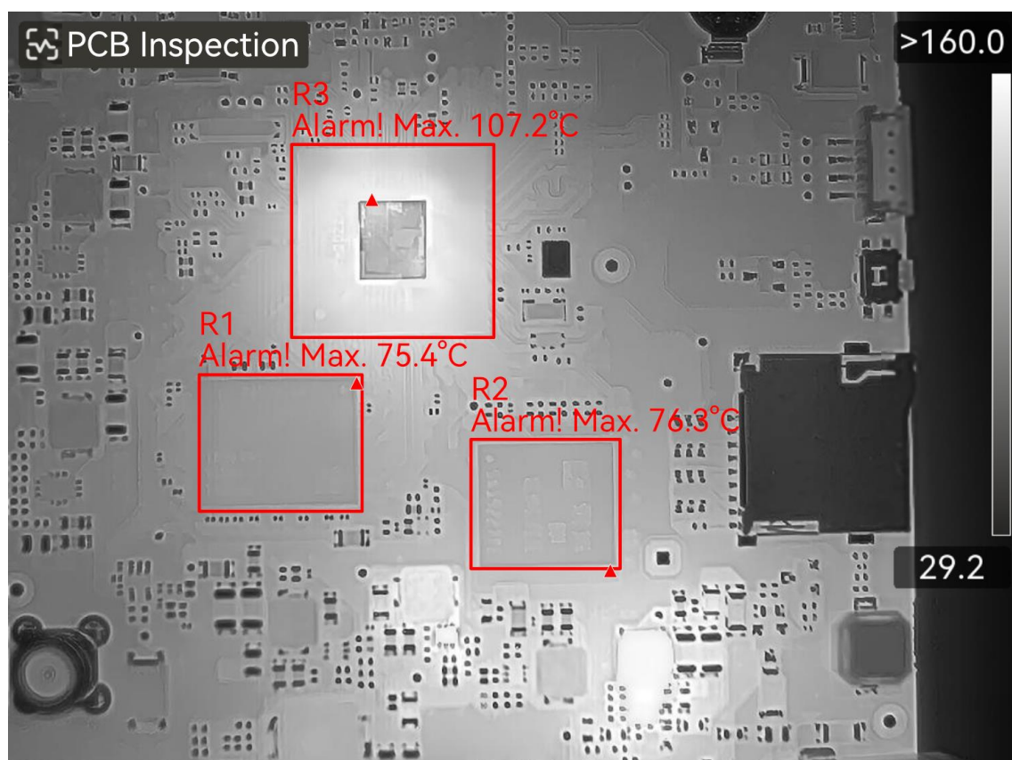
図5-1 PCB検査
