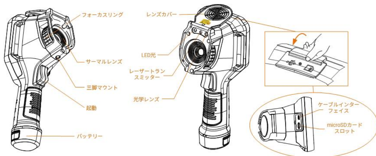
図 1-2 外観（側面図） I
