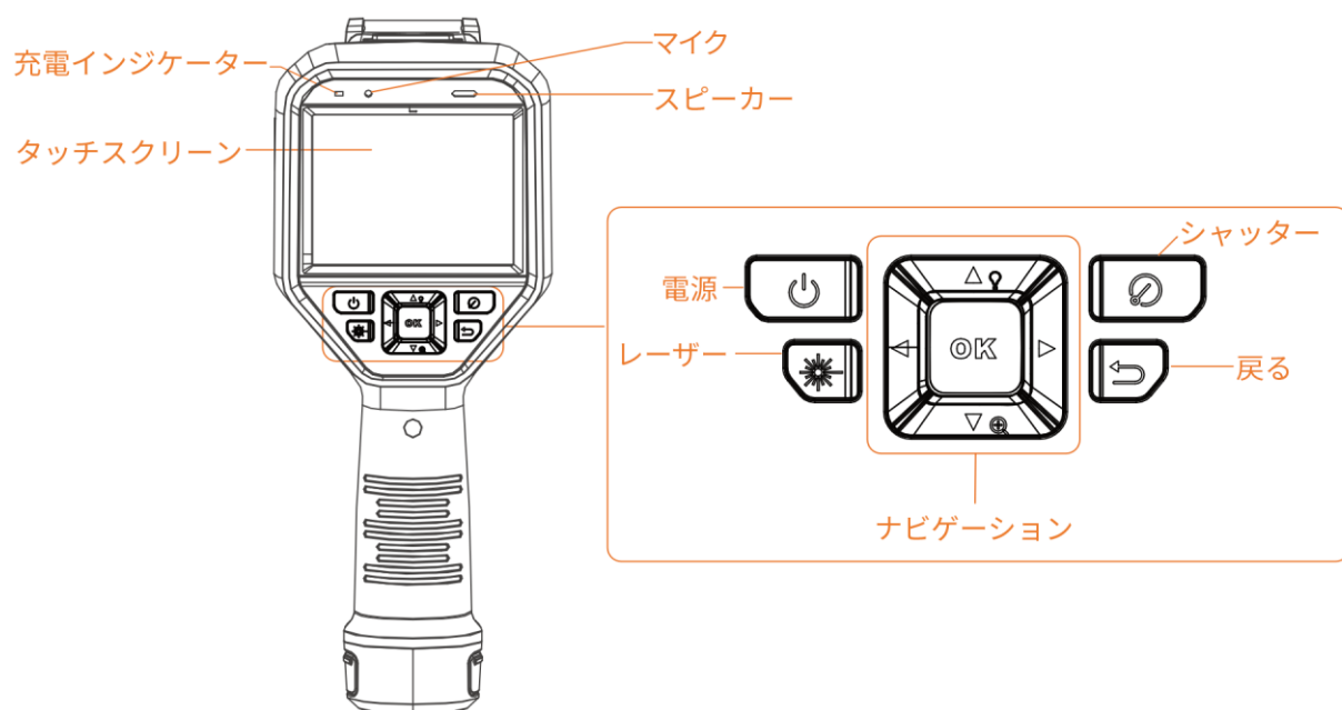
図1-1 外観（正面図）
